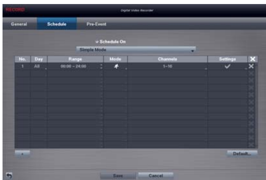
< Simple Mode >
